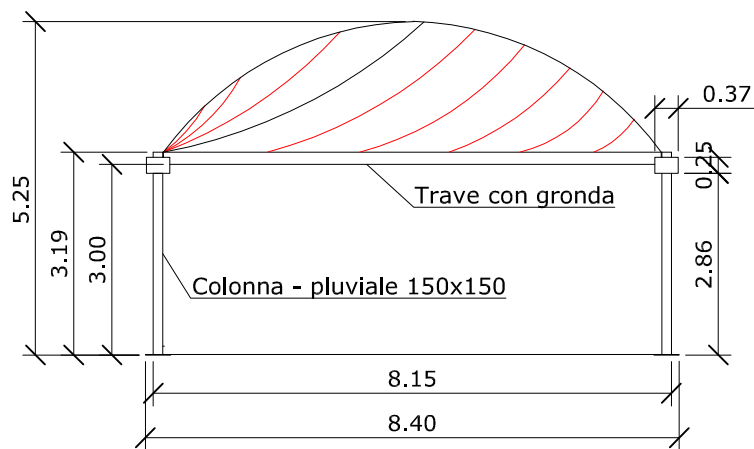
- PROSPETTO
