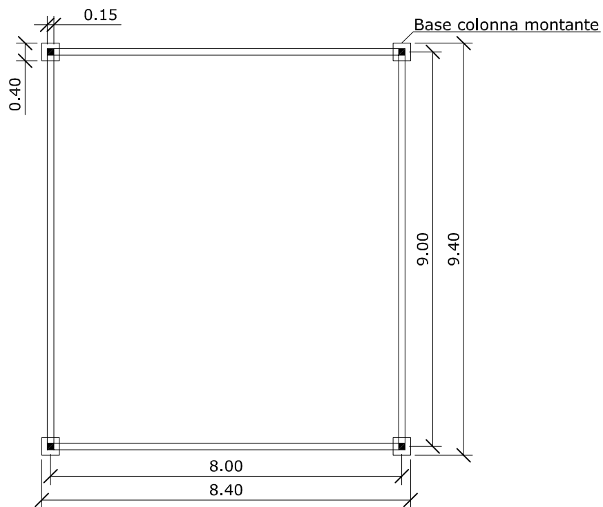
- PIANTA
